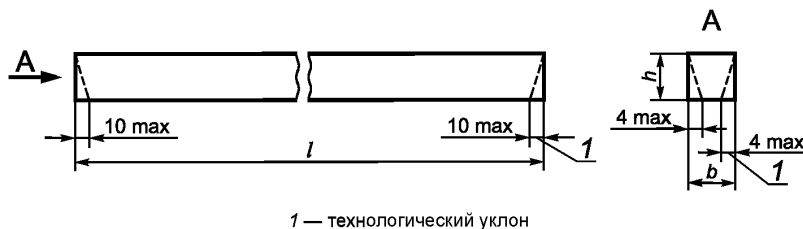
Рисунок 1 — Перемычка типа ПБ
