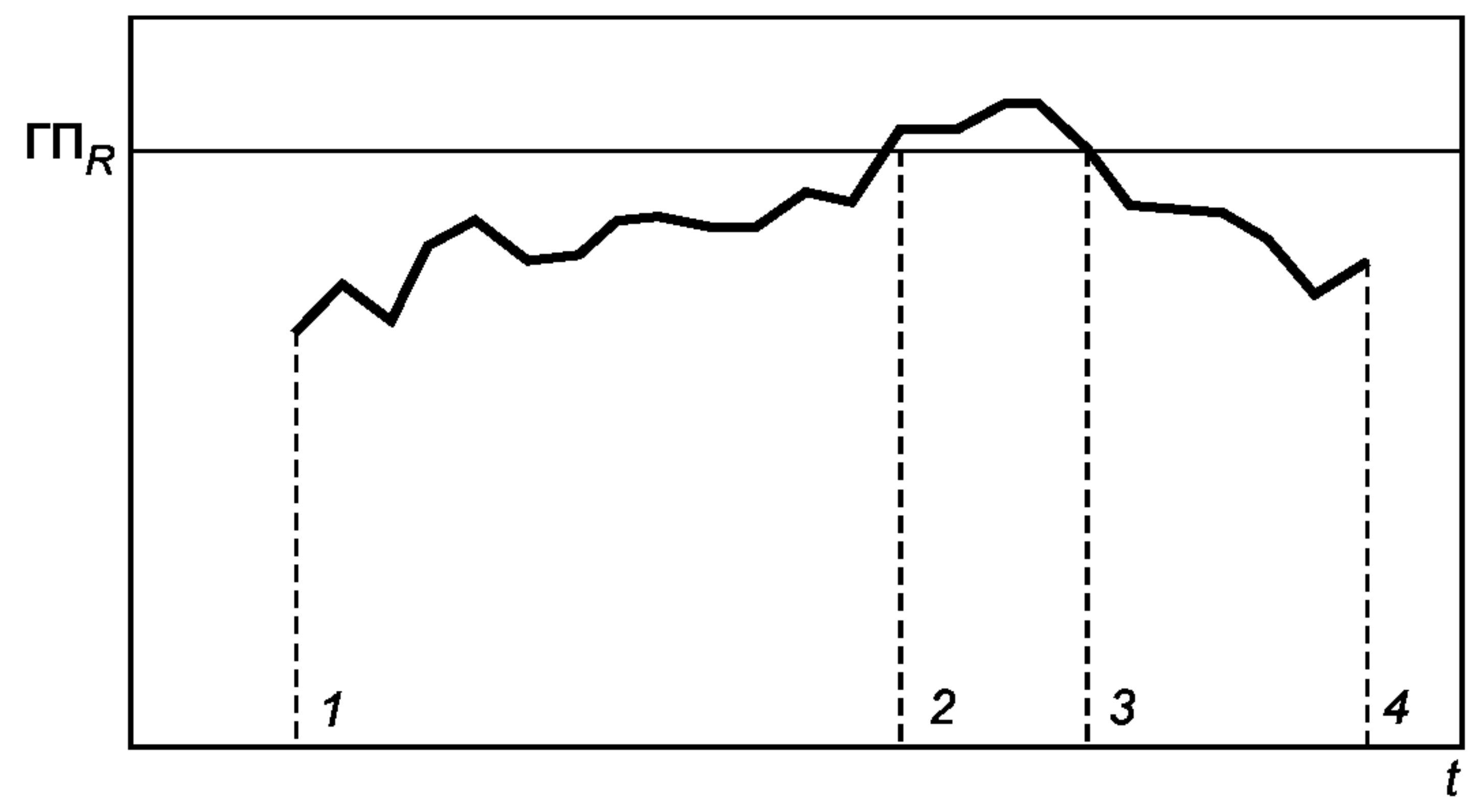
Рисунок Г.4 — Контрольная карта размахов
