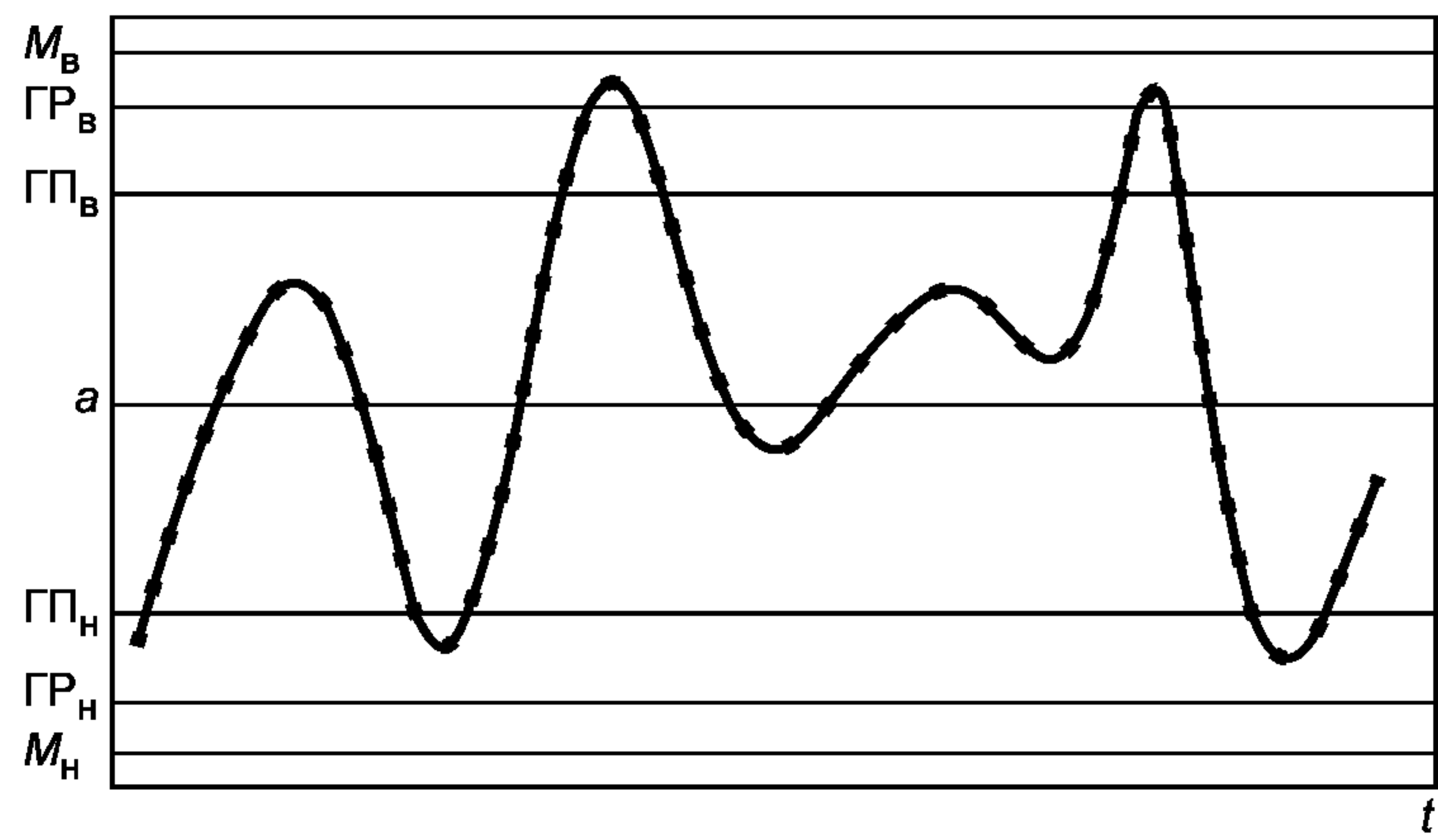
Рисунок Г.2 — Контрольная карта скользящих средних
