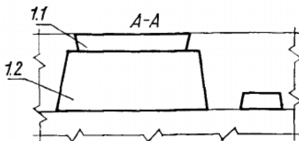
При формовании панели лицевой стороной вверх
