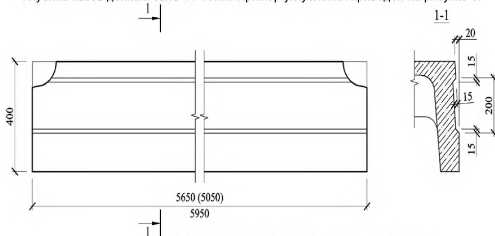
Рисунок 1 – Углубление на боковой поверхности плиты
