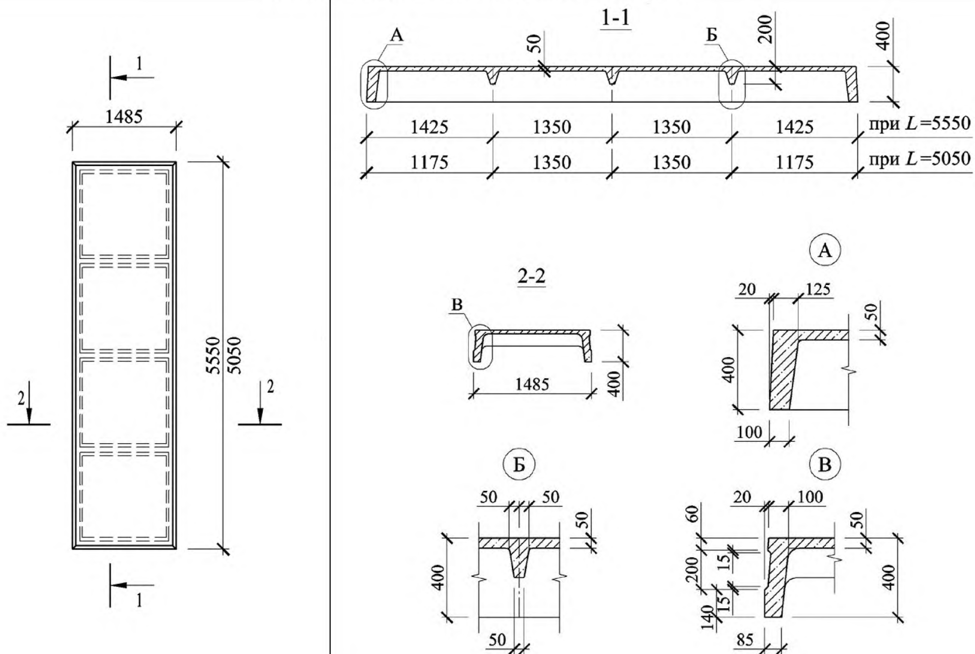
2 Плиты ряловые и межкопанные типоразмеров 1ПЗ и 1П4
