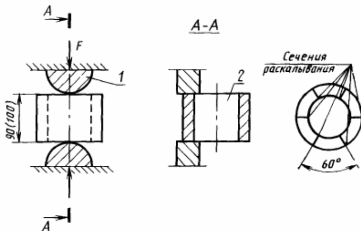
1—колющий полуцилиндр; 2—образец
