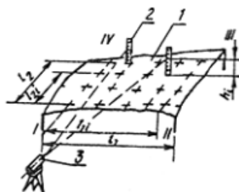
1 - проверяемая поверхность; 2 - линейка; 3 - нивелир
