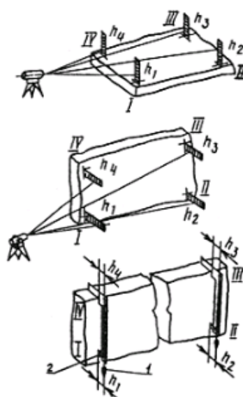
1 - отвес; 2 - шкала для отсчета
