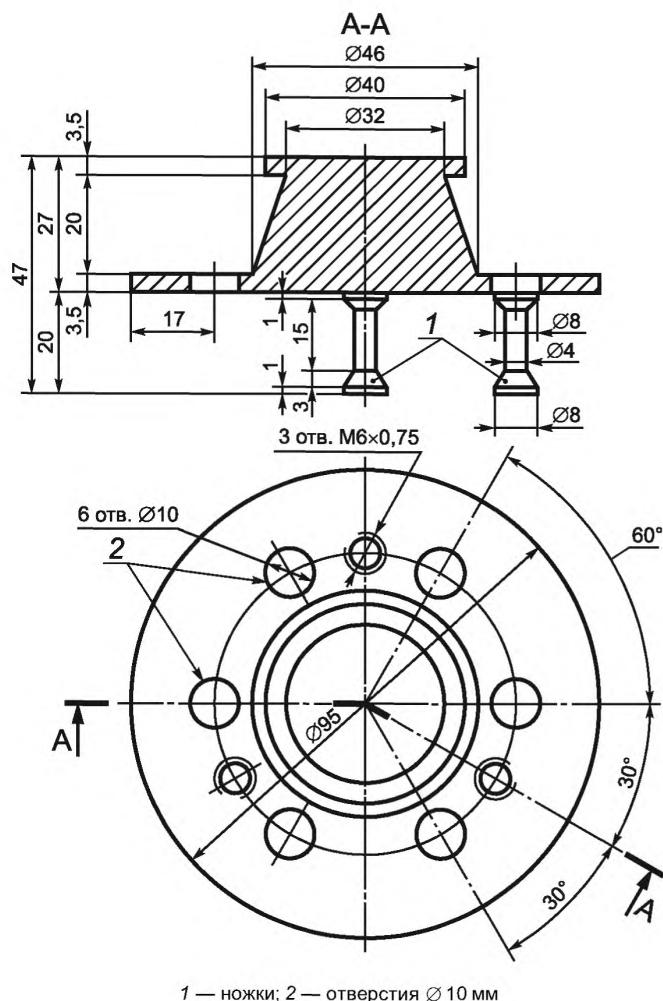
Рисунок 3 — Прибор Красного
